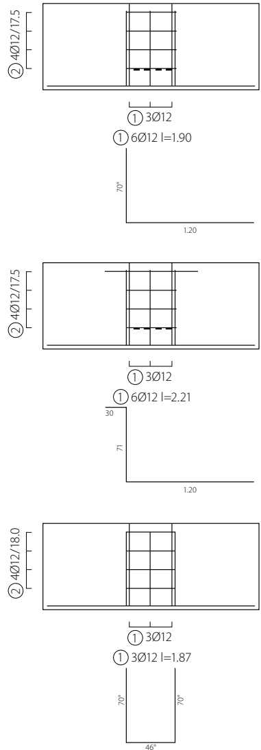
Beispiele Biegeformen Vertikalbügel
