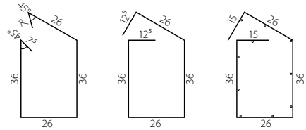
Biegeformen Rechteckbügel
