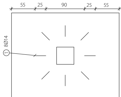
Draufsicht radiale Bügelanordnung
